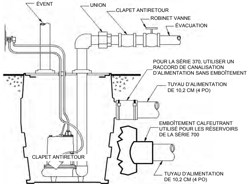
Fig. 2 – Installation type du système à une pompe Il s'agit d'une forme d'installation recommandée fournie à titre d'exemple. Les installations particulières peuvent varier.
